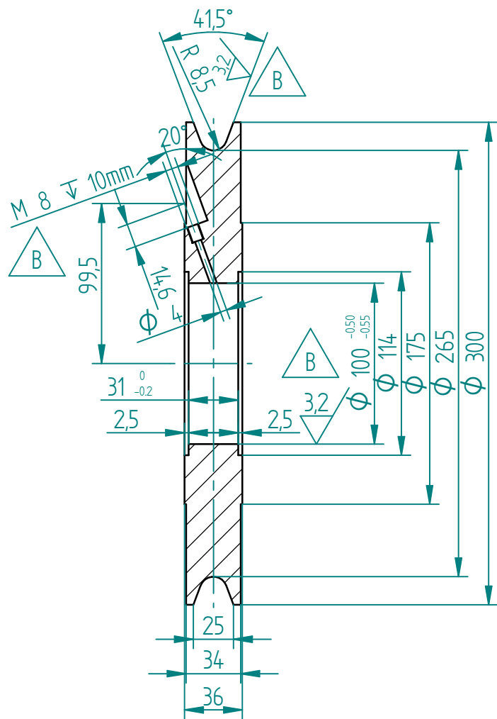
DOORSNEDE A-A
